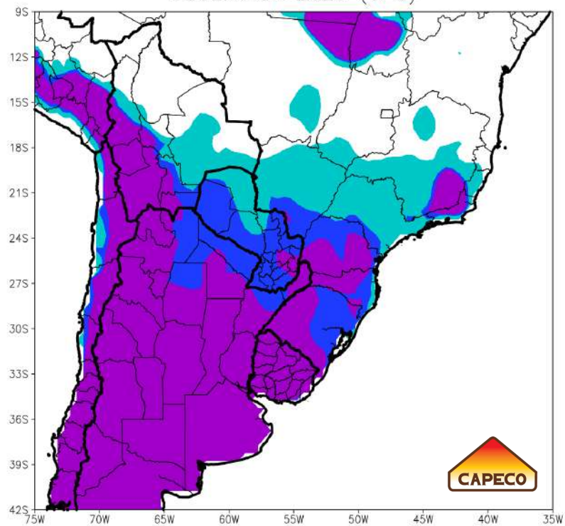
TEMPERATURA MINIMA ABSOLUTA ANUAL OBSERVADA 2025 (CPC)
