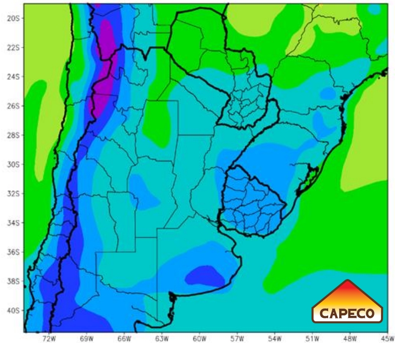
PERSPECTIVA DEL 15 AL 21 DE AGOSTO DE 2024 TEMPERATURA MINIMA(Grados Cent.)
