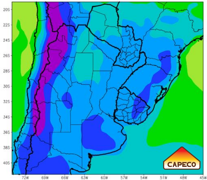
PERSPECTIVA DEL 8 AL 14 DE AGOSTO DE 2024 TEMPERATURA MINIMA(Grados Cent.)
