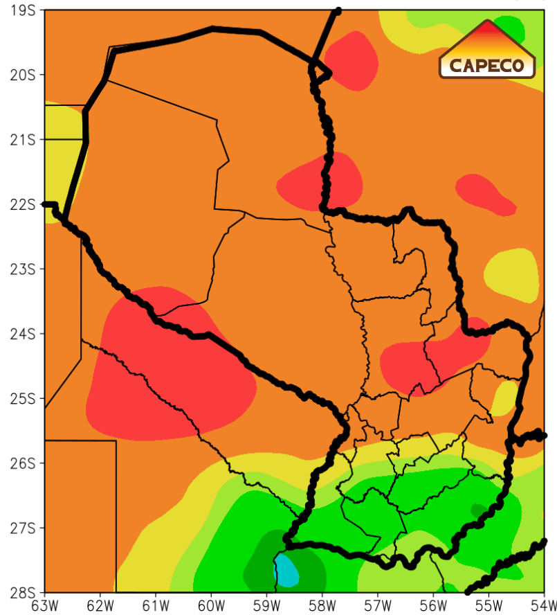
REANALISIS BHS AÑO 2024 MES 3 (Marzo) CONTENIDO DE AGUA DEL SUELO (%)
