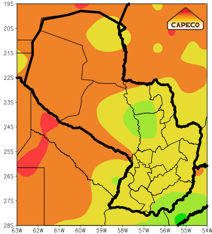
REANALISIS BHS AÑO 2024 MES 1 (Enero) CONTENIDO DE AGUA DEL SUELO (%)
