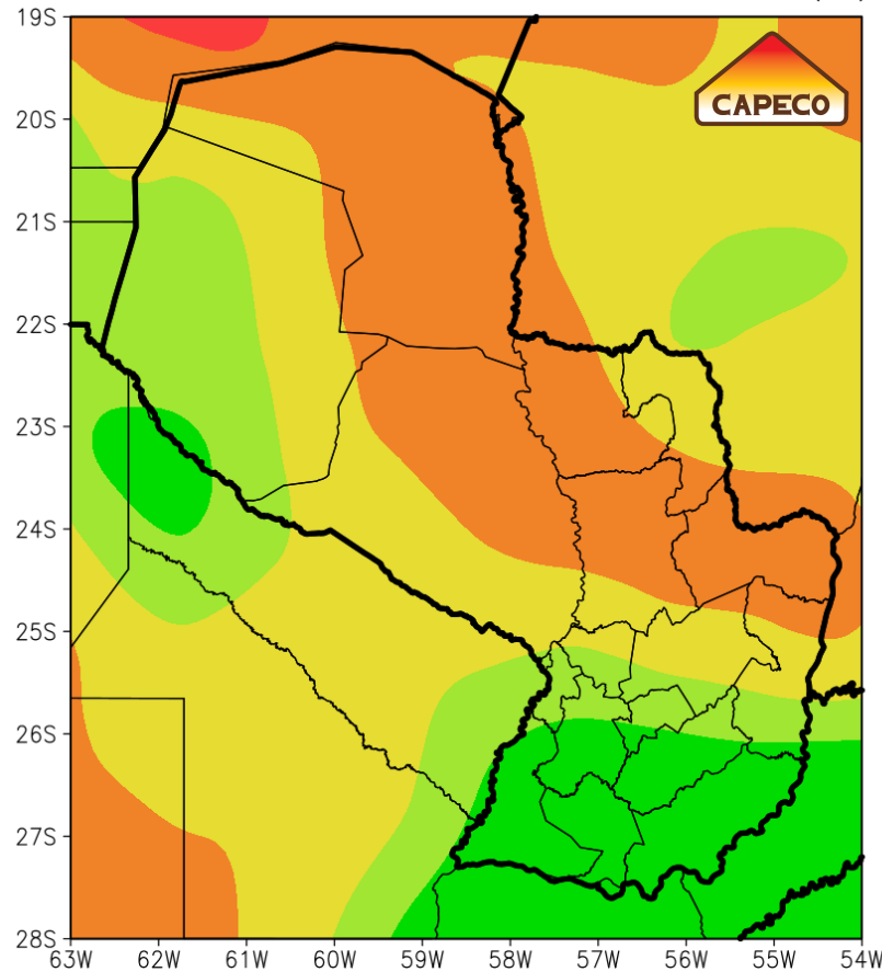
PRONOSTICO BHS AÑO 2024 MES 10 (Octubre) CONTENIDO DE AGUA DEL SUELO (%)
