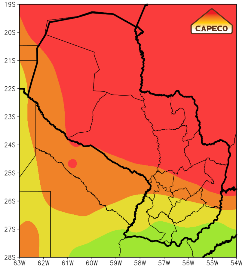
PRONOSTICO BHS ANO 2024 MES 6(Junio) CONTENIDO DE AGUA DEL SUELO (%)
