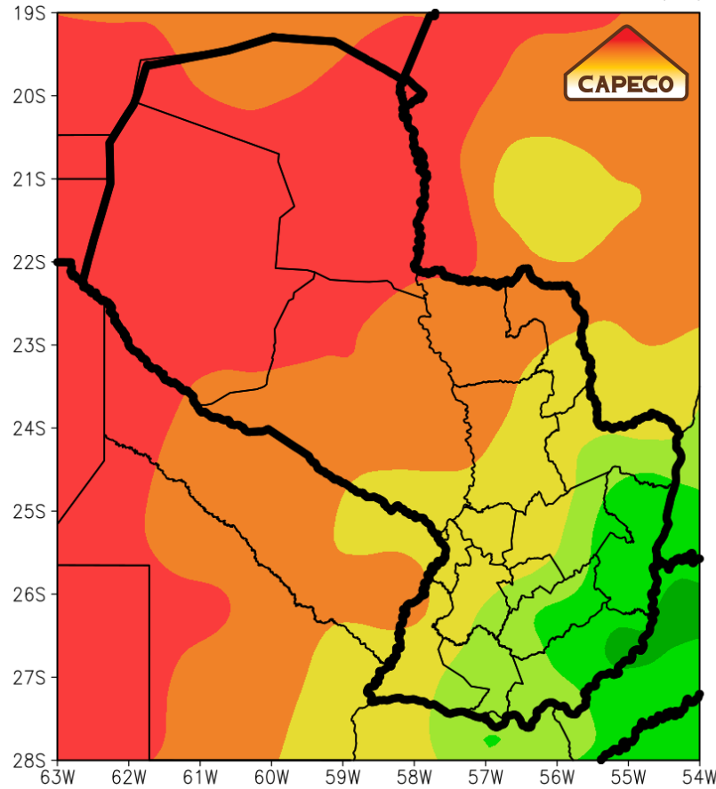
REANALISIS BHS AÑO 2023 MES 7 (Julio) CONTENIDO DE AGUA DEL SUELO (%)
