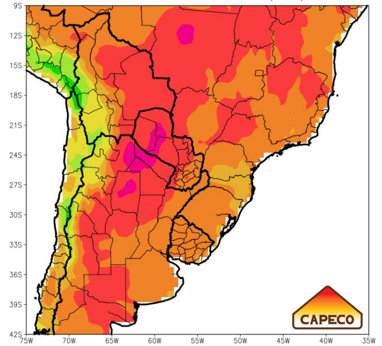
TEMPERATURA MAXIMA ABSOLUTA TEMPORADA 2023-2024 (CPC)
