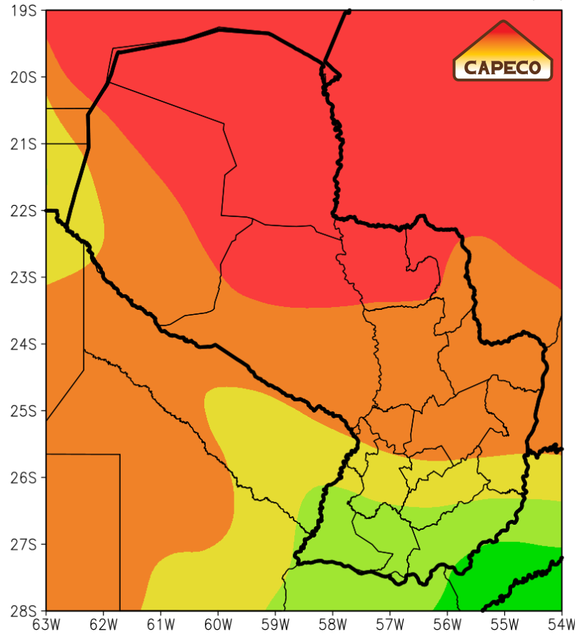
PRONOSTICO BHS ANO 2024 MES 9(Septiembre) CONTENIDO DE AGUA DEL SUELO (%)
