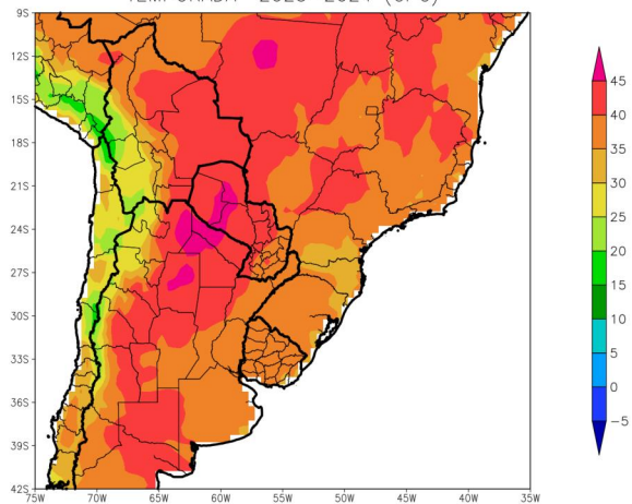
TEMPERATURA MAXIMA ABSOLUTA TEMPORADA 2023-2024 (CPC)
