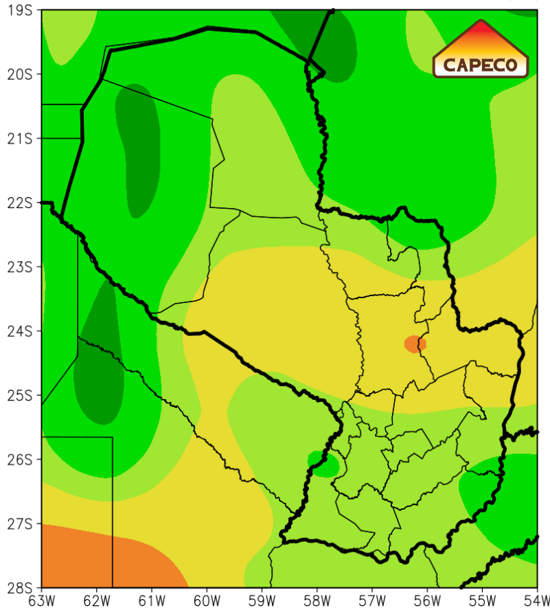
PRONOSTICO BHS AÑO 2024 MES 12 (Diciembre) CONTENIDO DE AGUA DEL SUELO (%)
