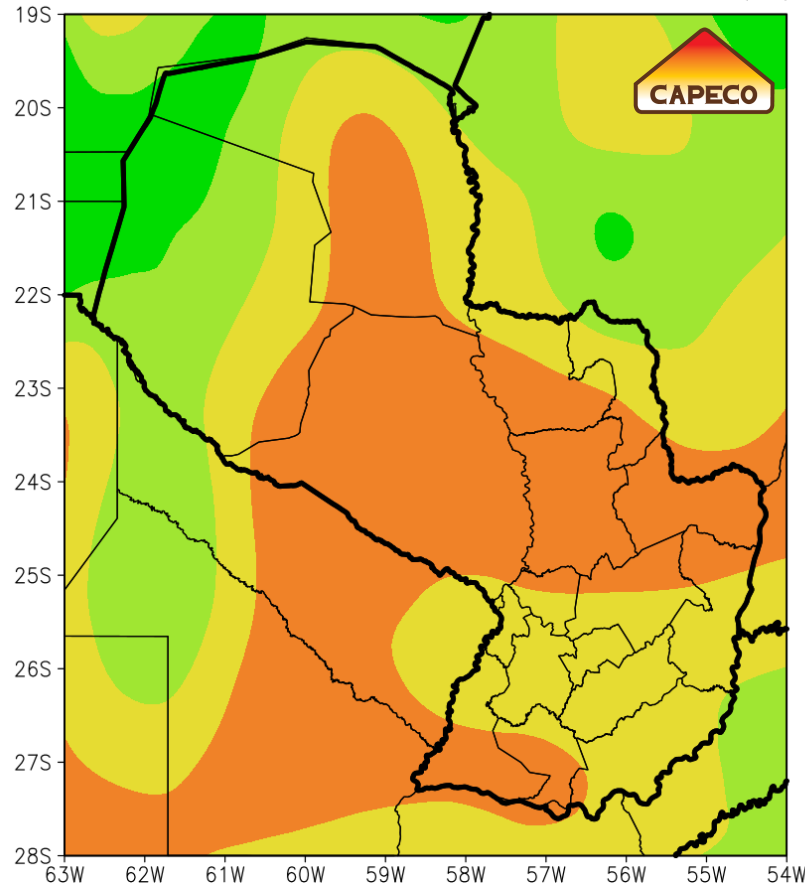
PRONOSTICO BHS ANO 2025 MES 1 (Enero) CONTENIDO DE AGUA DEL SUELO (%)
