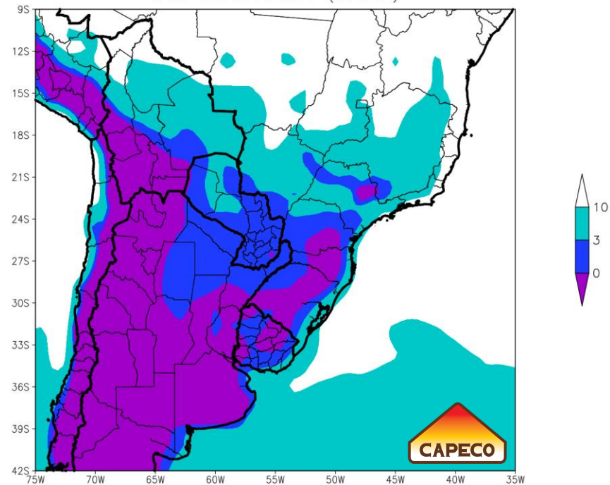
TEMPERATURA MINIMA ABSOLUTA PREVISTA TEMPORADA 2024 (CFSV2)
