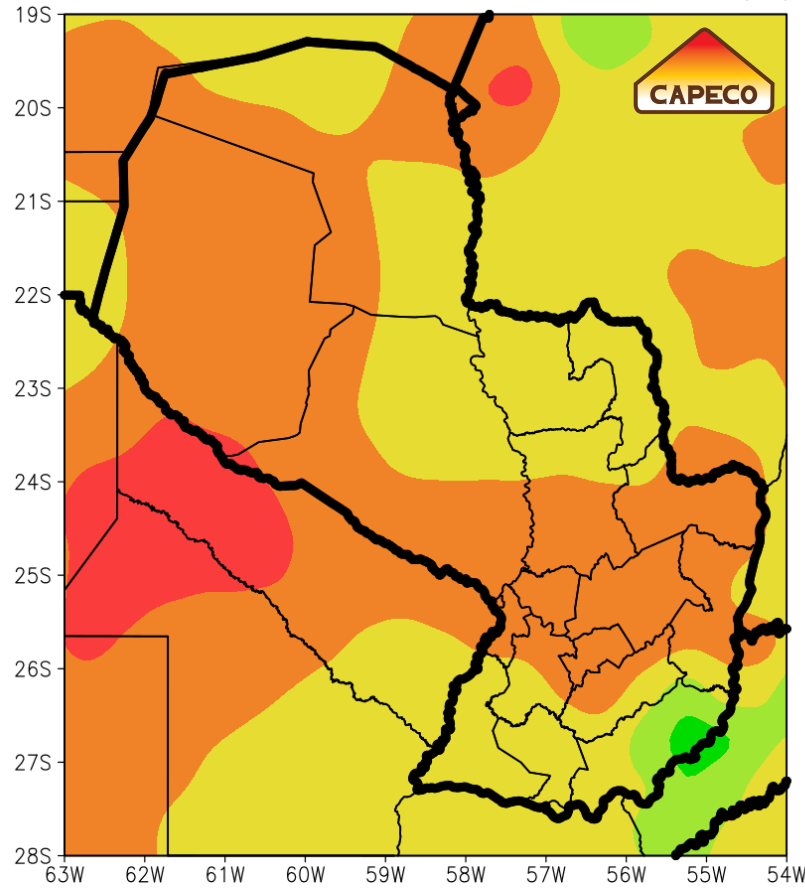
REANALISIS BHS AÑO 2024 MES 2 (Febrero) CONTENIDO DE AGUA DEL SUELO (%)
