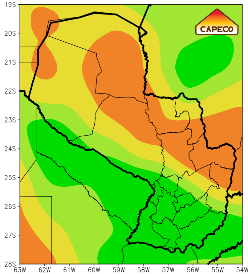
PRONOSTICO BHS ANO 2024 MES 11 (Noviembre) CONTENIDO DE AGUA DEL SUELO (%)
