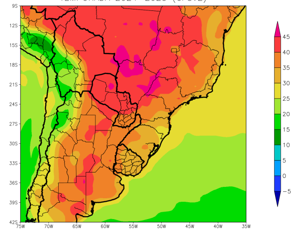
TEMPERATURA MAXIMA ABSOLUTA TEMPORADA 2024-2025 (CFSV2)
