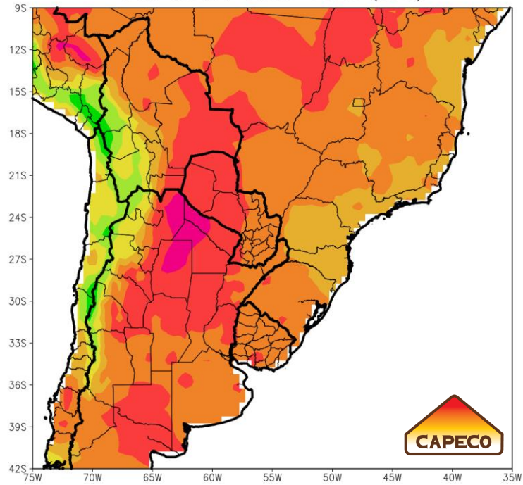
TEMPERATURA MAXIMA ABSOLUTA TEMPORADA 2022-2023 (CPC)
