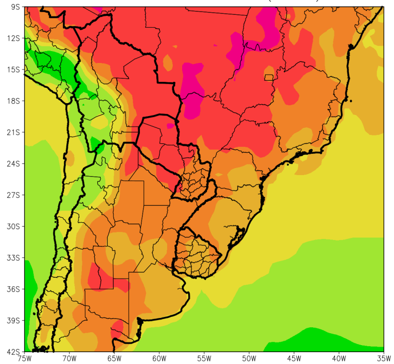
TEMPERATURA MAXIMA ABSOLUTA TEMPORADA 2023-2024 (CFSV2)
