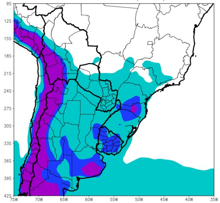
TEMPERATURA MINIMA ABSOLUTA TEMPORADA 2023 (CFSV2)
