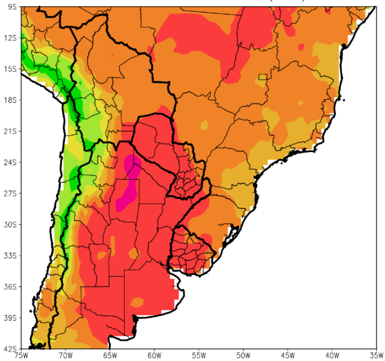
TEMPERATURA MAXIMA ABSOLUTA TEMPORADA 2021-2022 (CPC)
